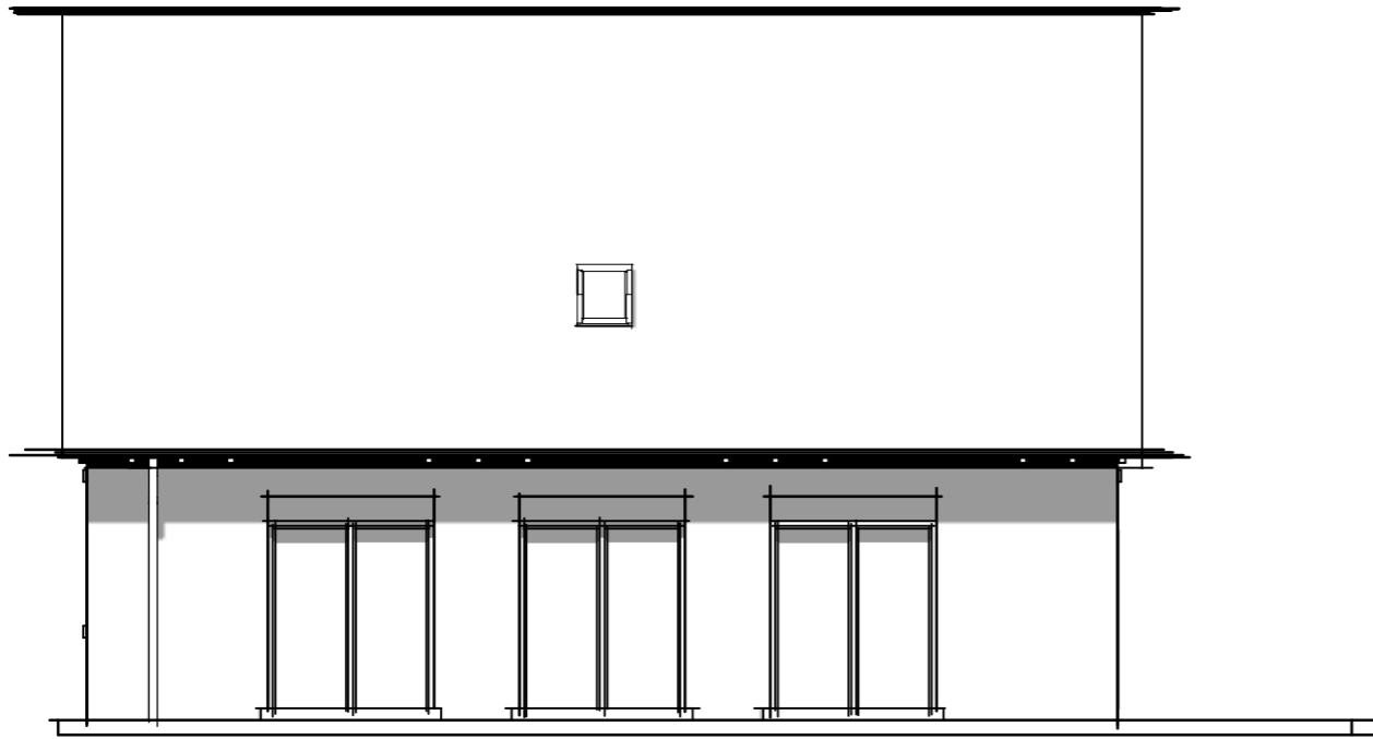
Ansicht Westen
